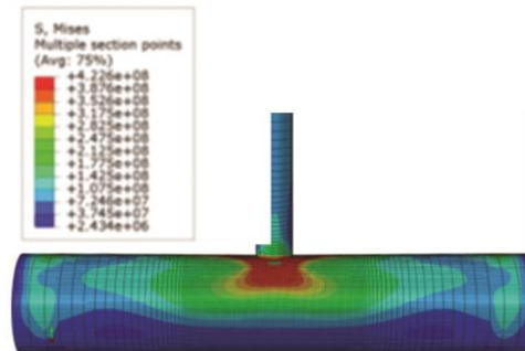
شکل (۴) شکل تغییر فرم یافته برای حالت تقویت ۸ لایه FRP
