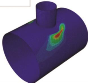
شکل (۷) گسیختگی ناشی از کشش الیاف
