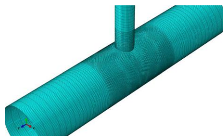
شکل (۱) نمونه ای از مدل اتصال
